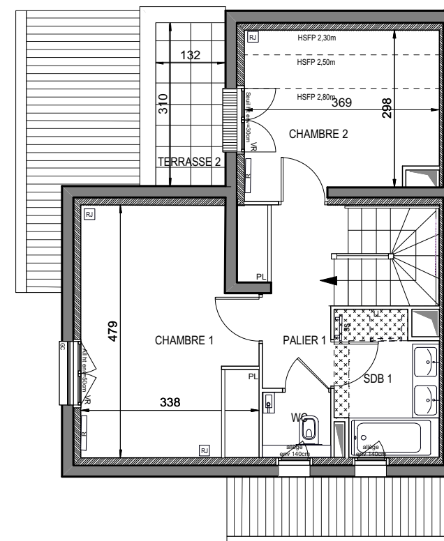
1er ETAGE
