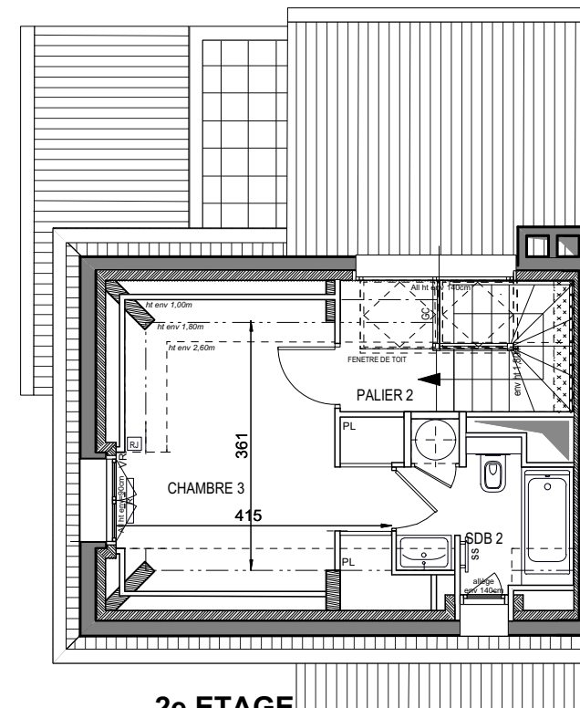
2e ETAGE
